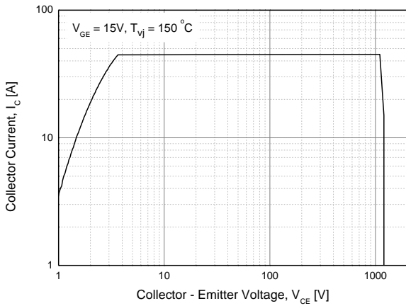
Fig. 15 RBSOA
