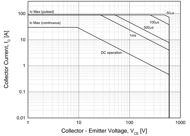
Fig. 14 SOA
